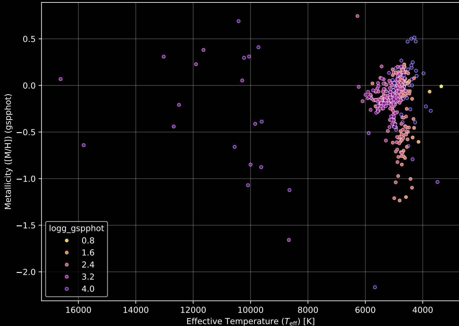
APOGEE DR17 Field: [120-08] Stellar Population Parameters (n= 433)
